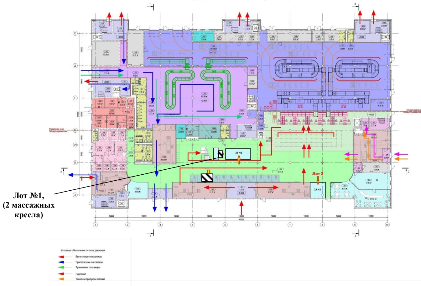
План функционального зонирования 1-го этажа (на отм. 0.000)
